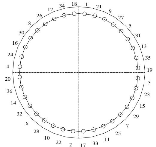
36 BOLT
