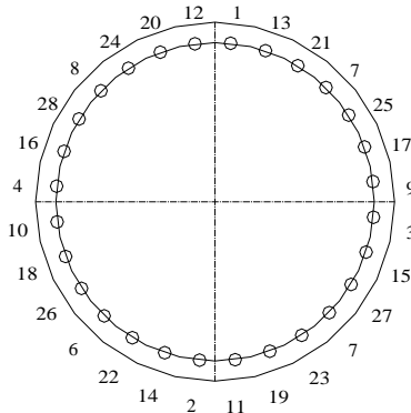
28 BOLT
