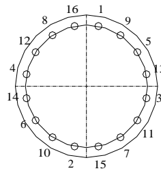
16 BOLT
