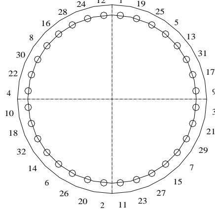
32 BOLT
